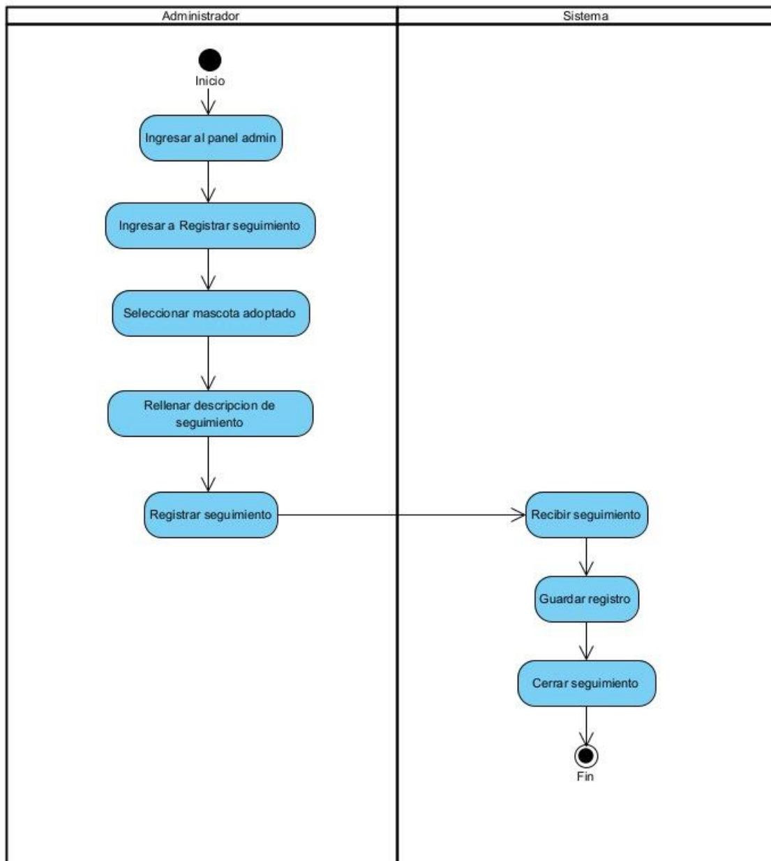
Diagrama de proceso de Seguimiento de Adopción
