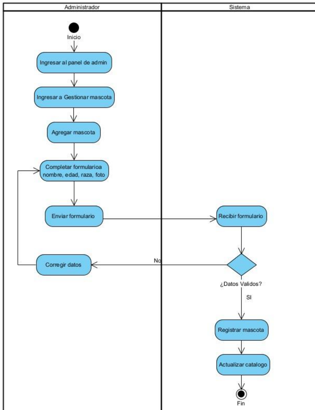
Diagrama de proceso de Agregar Mascota
