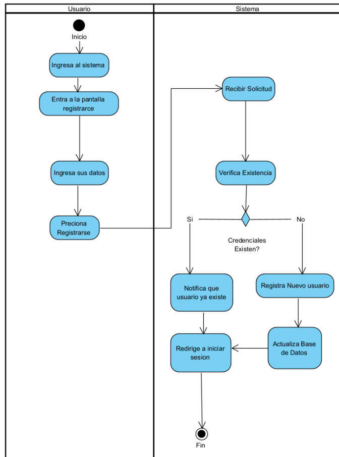
Diagrama de proceso de Registro de Usuario
