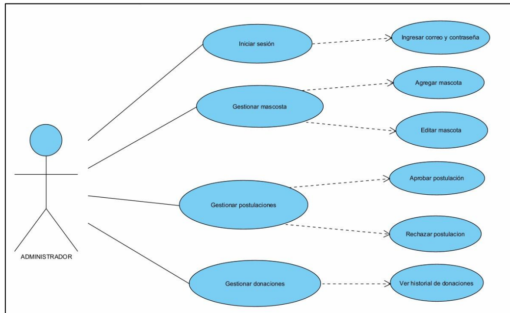
Diagrama de casos de uso para el Administrador
