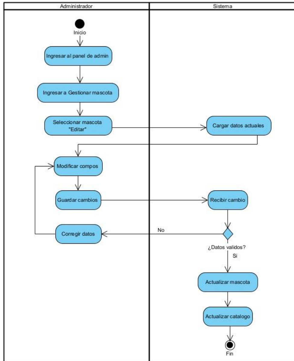
Diagrama de proceso de Editar Mascota
